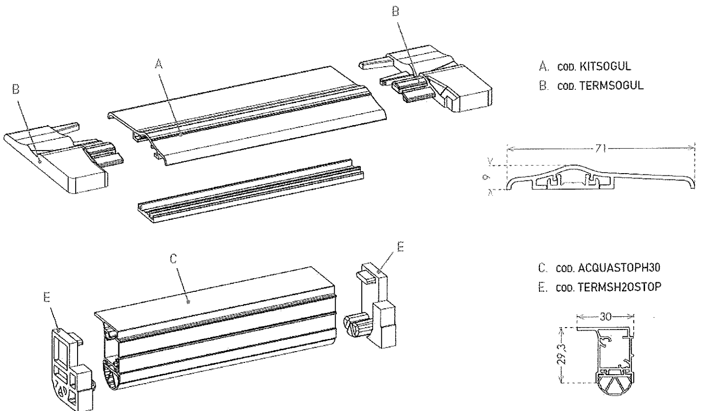
Fig. 6: Dettaglio soglia del campione sottoposto a prova (dimensioni nominali dichiarate, espresse in mm.)
