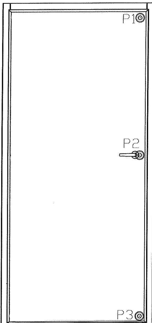
Fig. 7. Assetto sperimentale prova di resistenza al carico del vento vista interna: (schema di posizionamento dei trasduttori)
