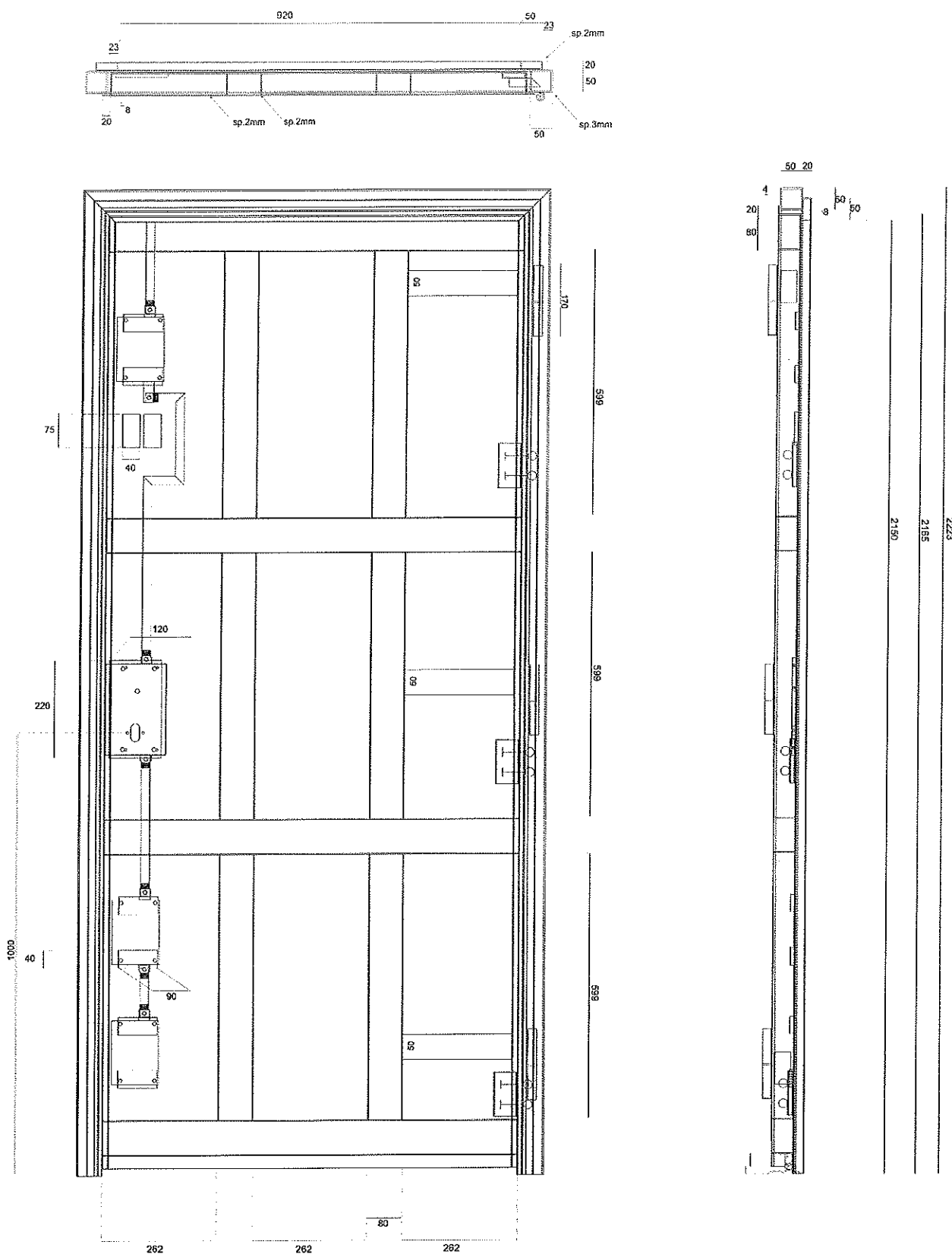
Fig. 1: Prospetto e sezioni del campione sottoposto a prova (dimensioni nominali dichiarate, espresse in mm)
