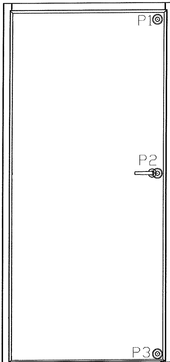
Fig. 6. Assetto sperimentale prova di resistenza al carico del vento vista interna: (schema di posizionamento dei trasduttori)
