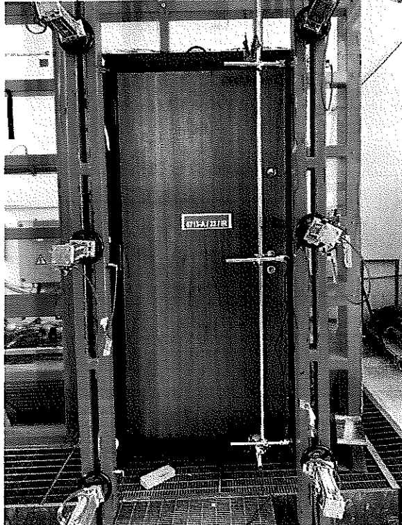
Foto 2: Campione sottoposto a prova durante i test di resistenza al carico del vento
